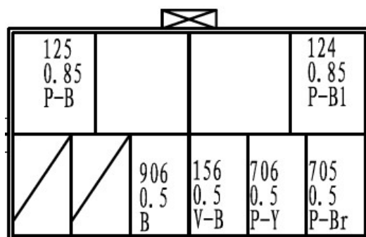
左前门中控锁
