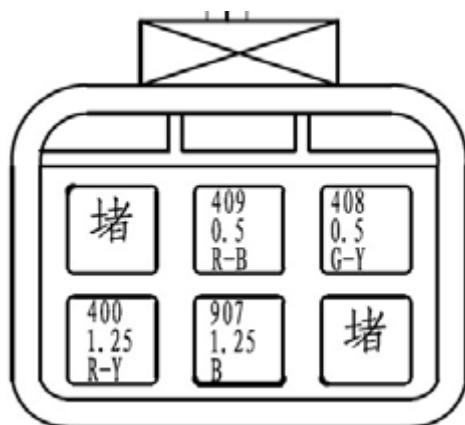
左前门升降电机
