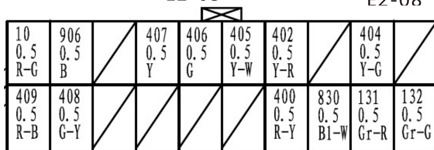
左前门窗开关
