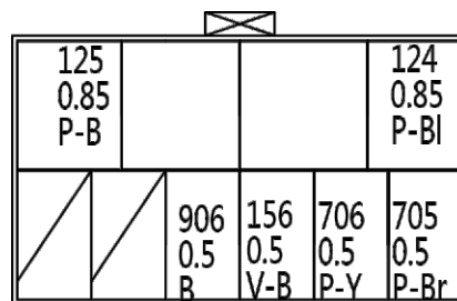
左前门中控锁
