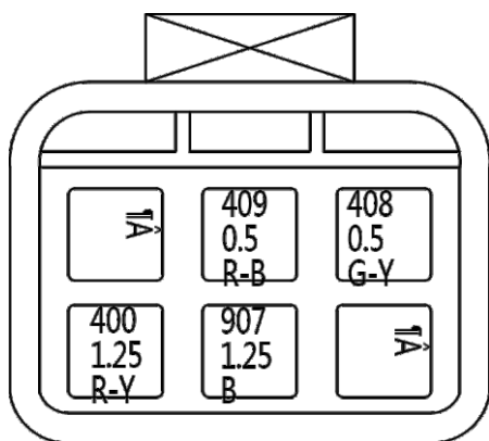
左前门升降电机
