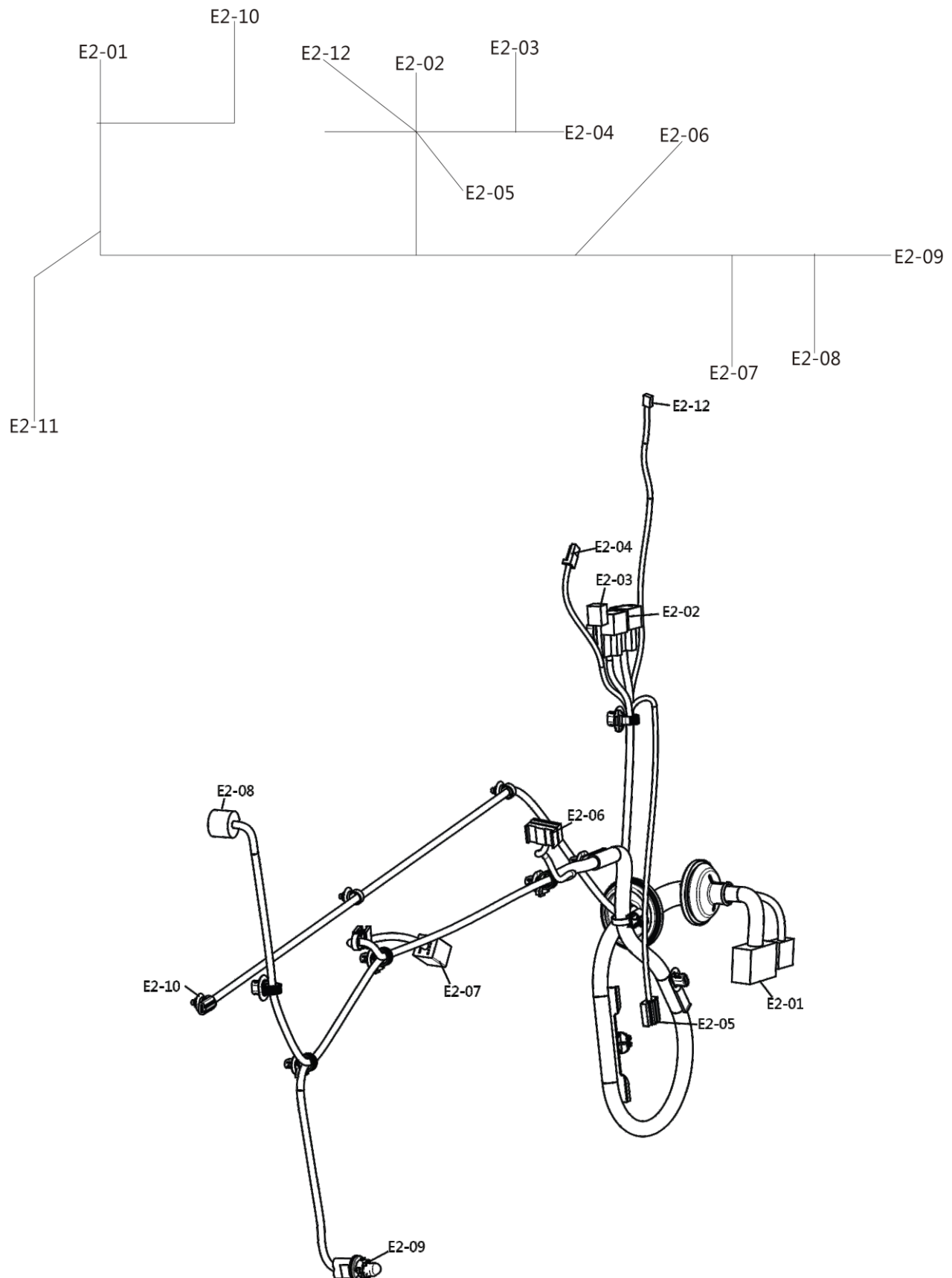
线束连接图
