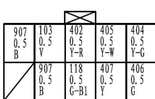
接左侧电动后视镜
